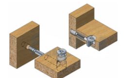
Соединение деталей эксцентриковыми стяжками
